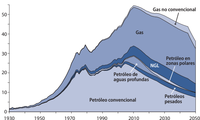
FIGURA 2: PROYECCIÓN DE ASPO SOBRE EL CENIT DE PETRÓLEO Y GAS
